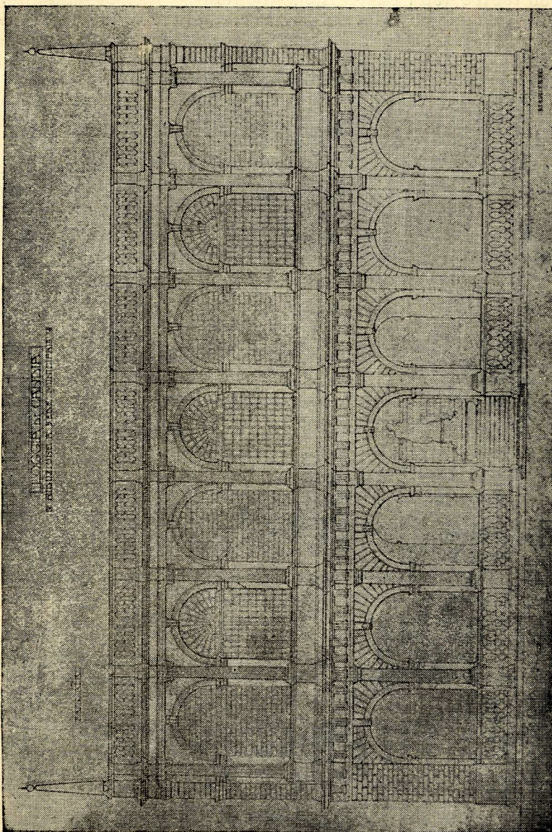
Εἰκ. 25. Σχέδιον προόψεως ἀναστηλώσεως τῆς Λότζας, ὑπὸ τοῦ Ongaro.
